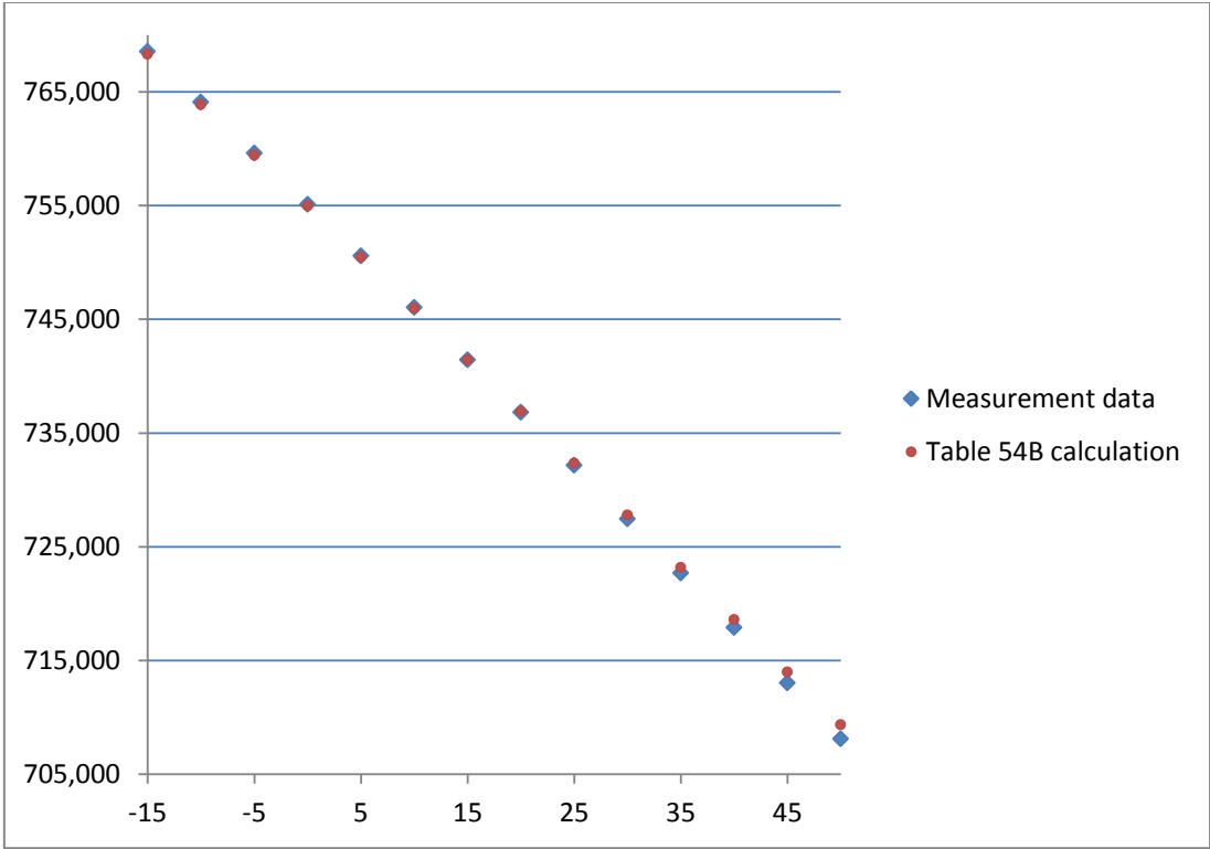
Example 3: SSR 3.43 (kg/m 3 ) 2 - E10 (Winter, Super)
